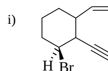
(S)-1-bromo-3-ethenyl-2-ethynylcyclohexane
