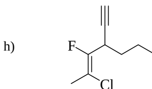
E-2-chloro-3-fluoro-4-propyl-2-hexen-5-yne
