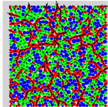
■ Stress Map
