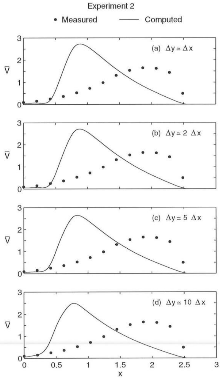
Figure 4.10: Sensitivity analysis for experiment 2 with (a) \Delta y \simeq \Delta x , (b) \Delta y \simeq 2\Delta x , (c) \Delta y \simeq 5\Delta x , (d) \Delta y \simeq 10\Delta x .
